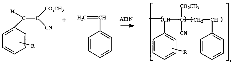
Scheme 1. ST-TSE copolymer synthesis. R = 2,3-, 2,4-, 2,5-, 3,4-, 3,5-dimethoxy, and 3-ethoxy-4-methoxy.
